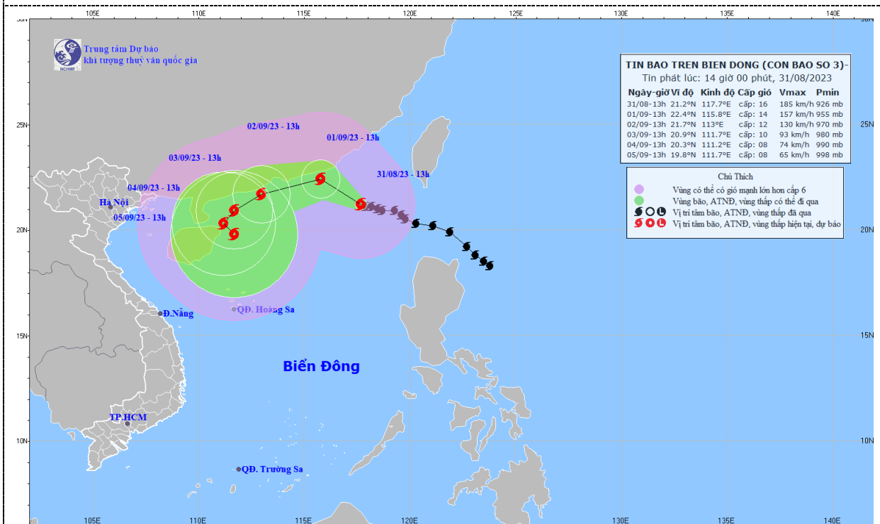
Hình 1. Bản đồ dự báo quỹ đạo và cường độ bão số 3 phát lúc 14h00 ngày 31/8/2023
